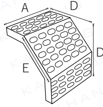
Internal Bend 內曲型
