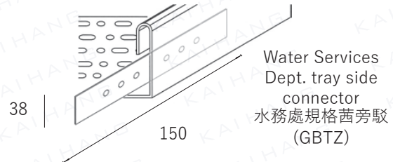
Common Type 普通款 (DBC)
