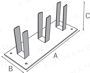
Cable support 電線掛片
