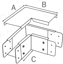
Front opening 正面蓋型
