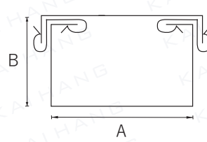
Clip Fix 彈夾蓋型
