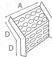
External Bend 外曲型
